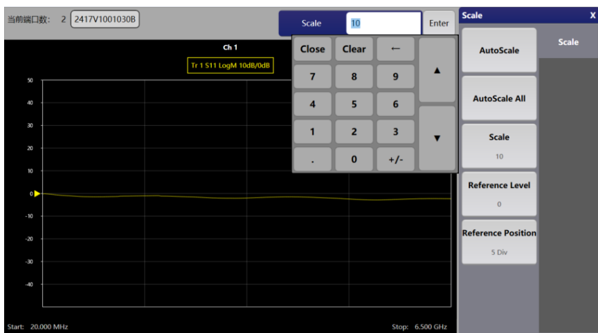
图 18 纵坐标刻度及扩展功能区图
