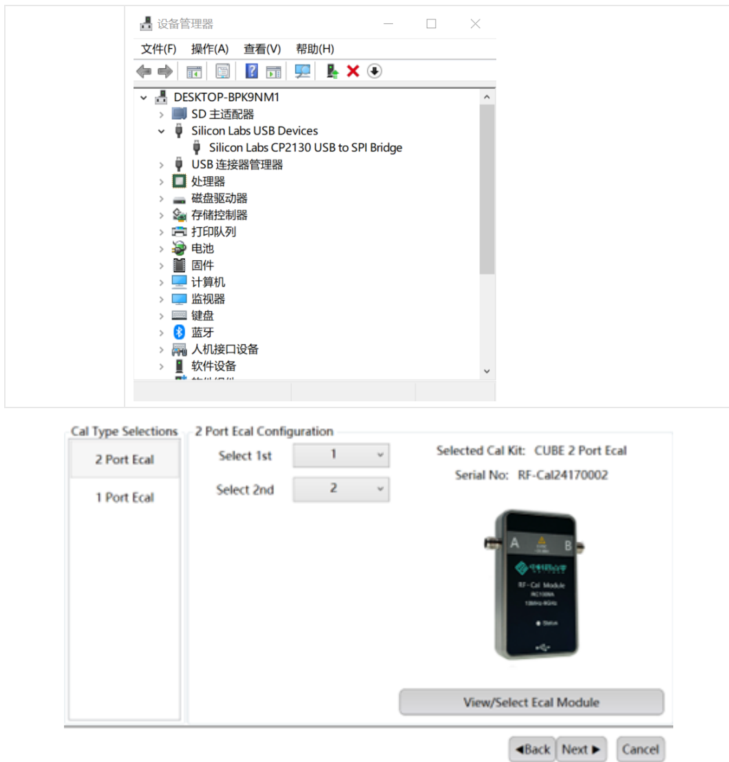
图 27 电子校准及扩展功能区图
