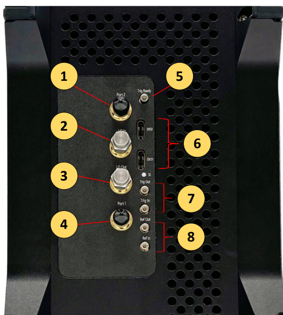
图 2. 左面板布局图
