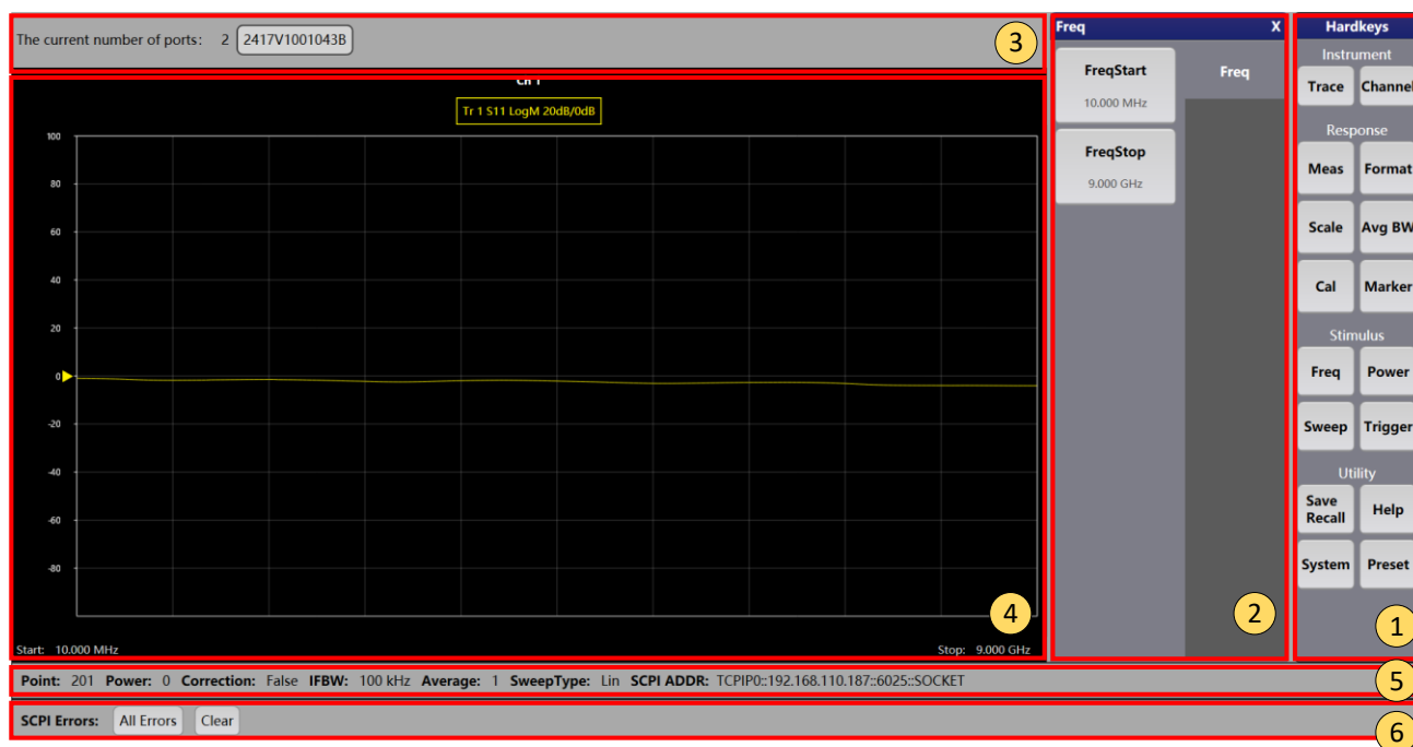
图 1 主界面功能区
